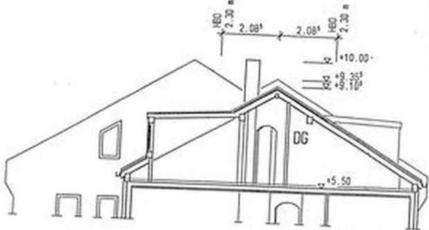
SCHNITT C-C
