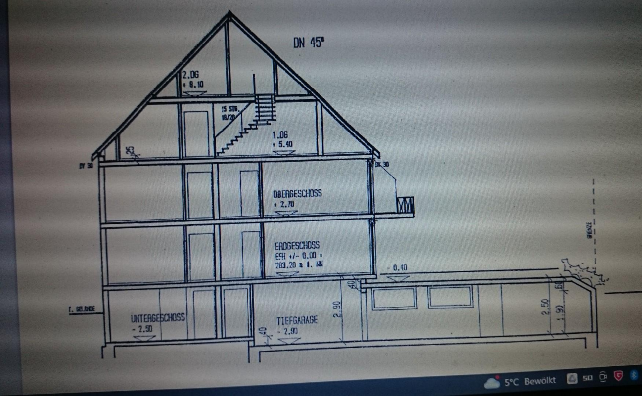
Schnittdarstellung Haus
