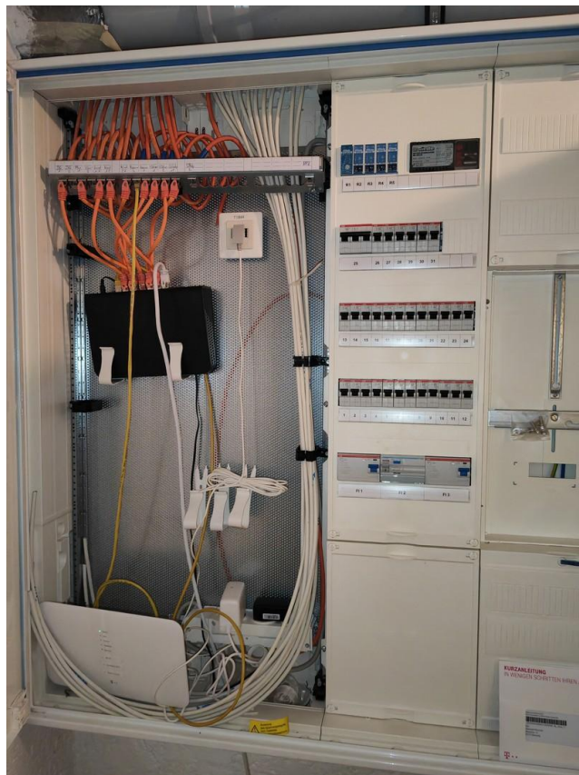
Schaltkasten UG
