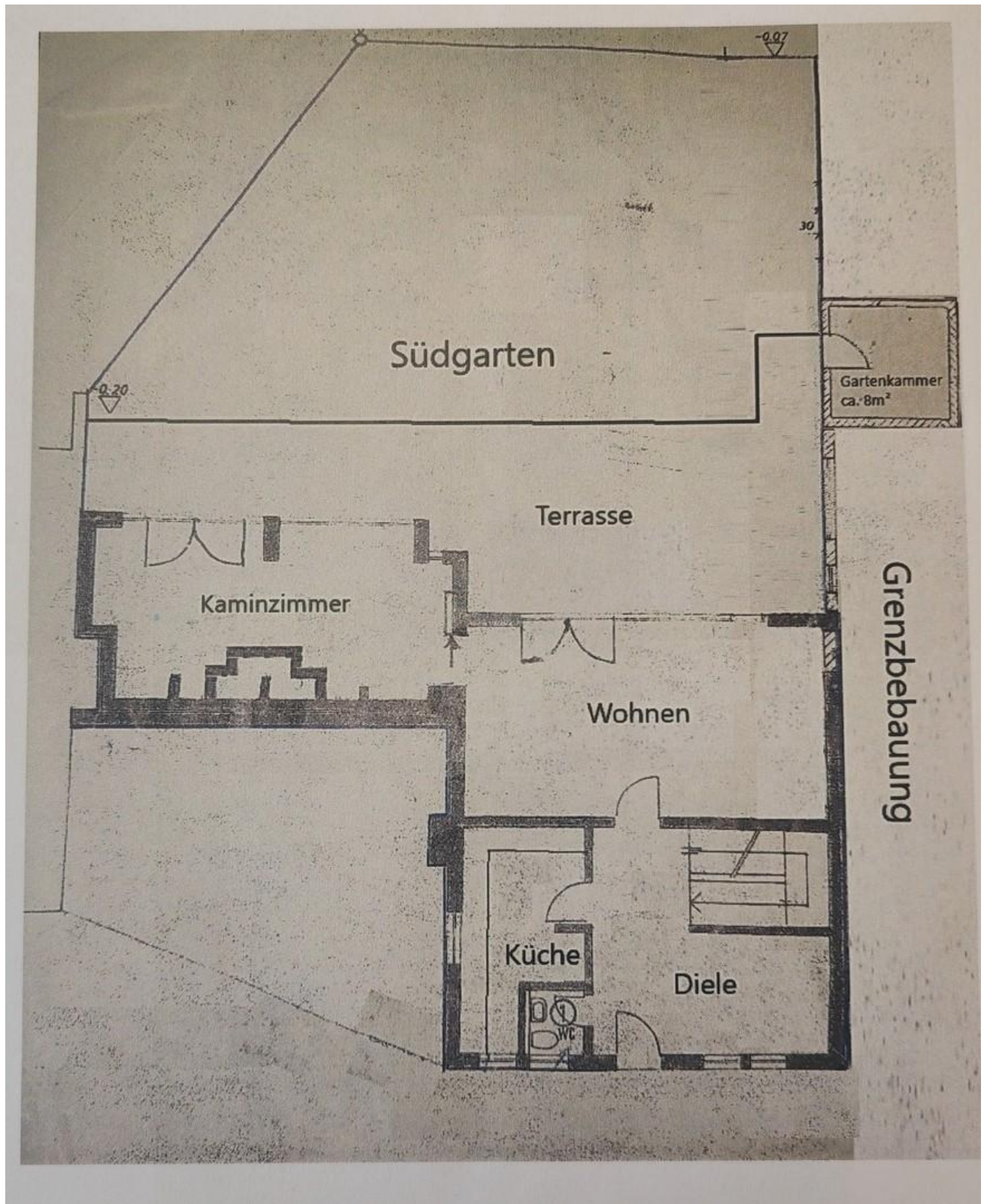
Grundriss EG mit Gartenhaus
