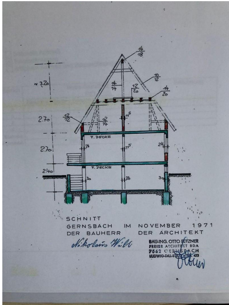
Schnitt des Hauses
