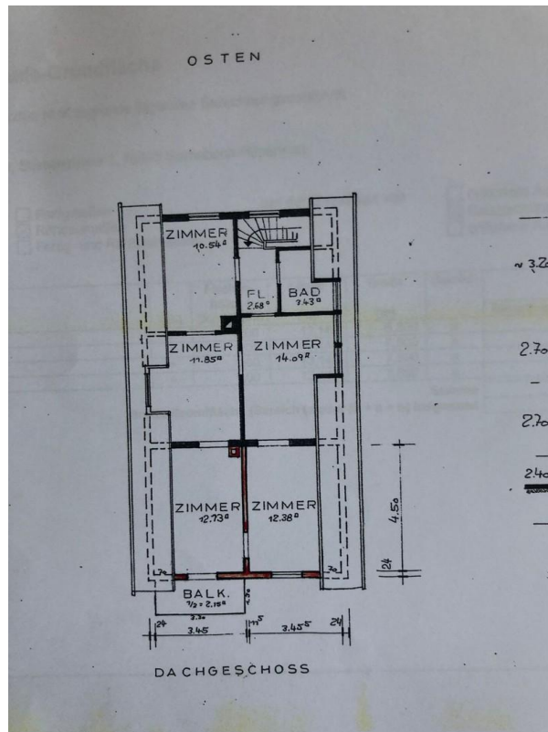
Grundriss DG
