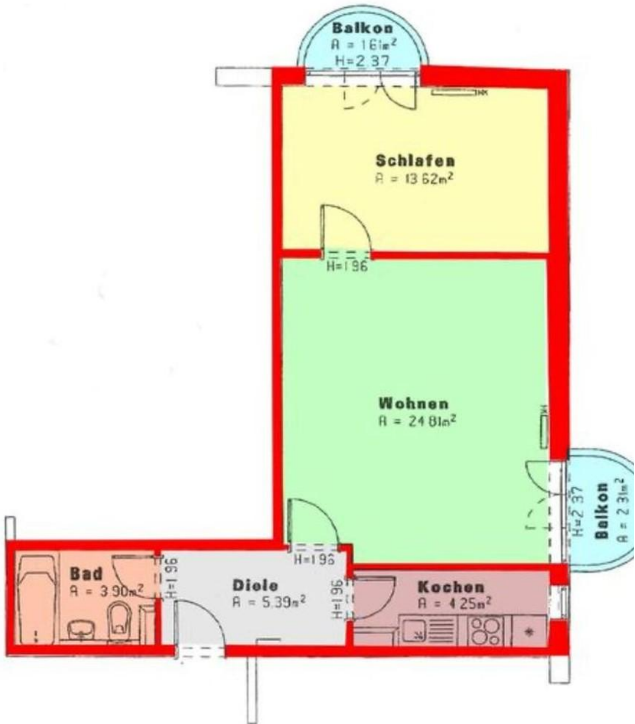
Grundriss
