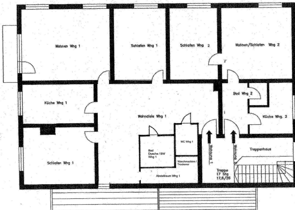
Grundriss Wohnung 2
