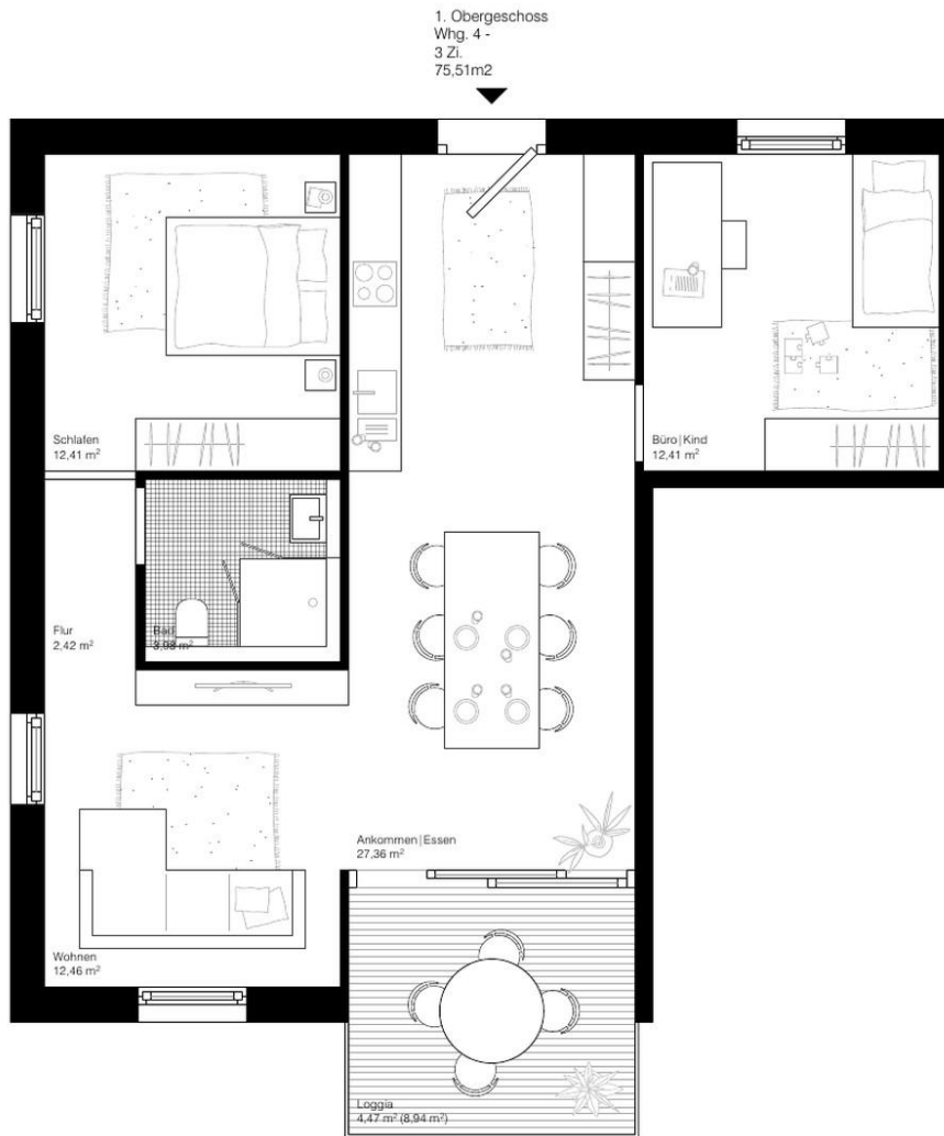
Grundriss Whg. 4
