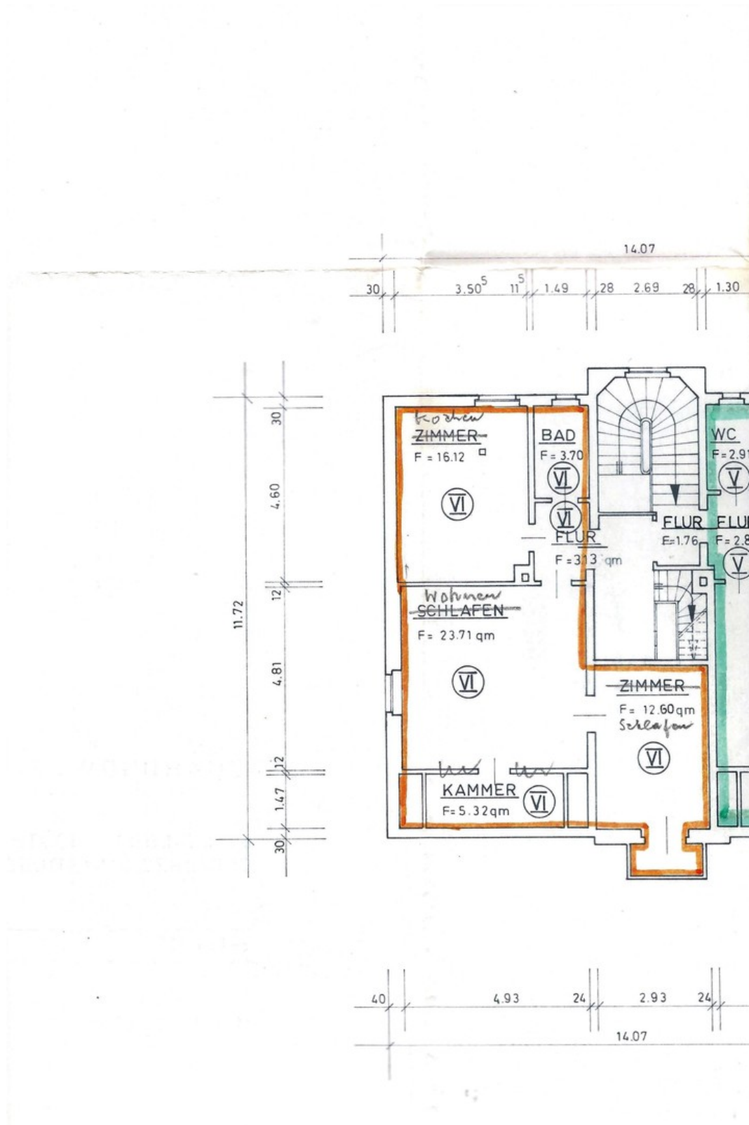
Grundriss DG
