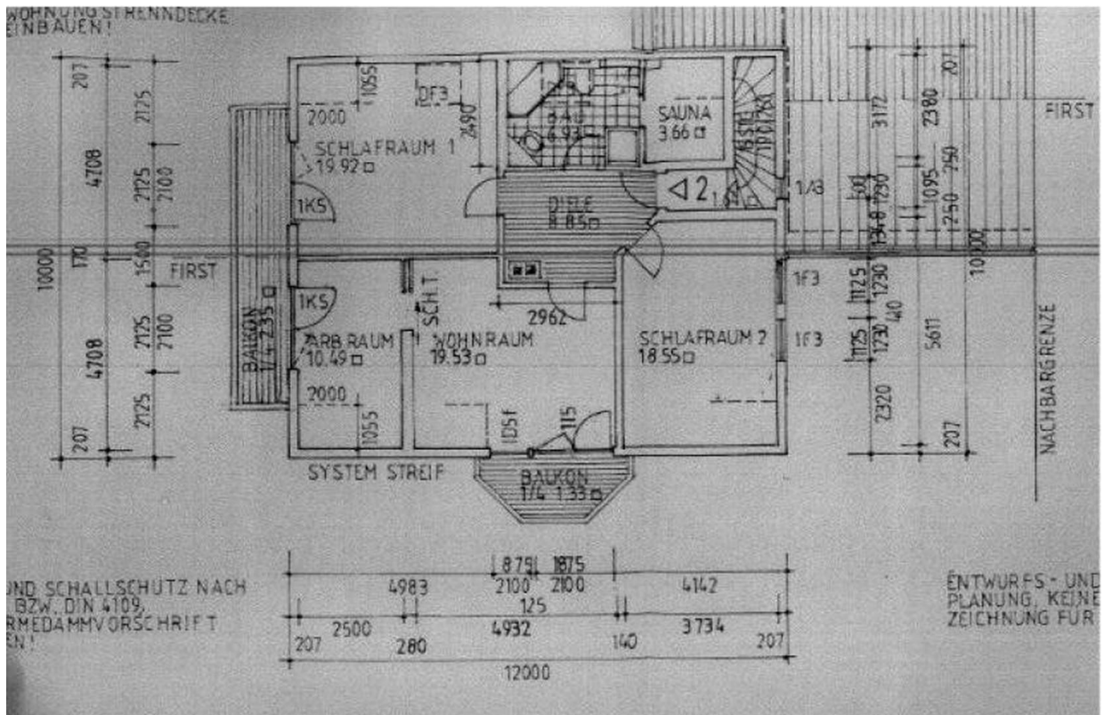
Grundriss Dachgeschoss
