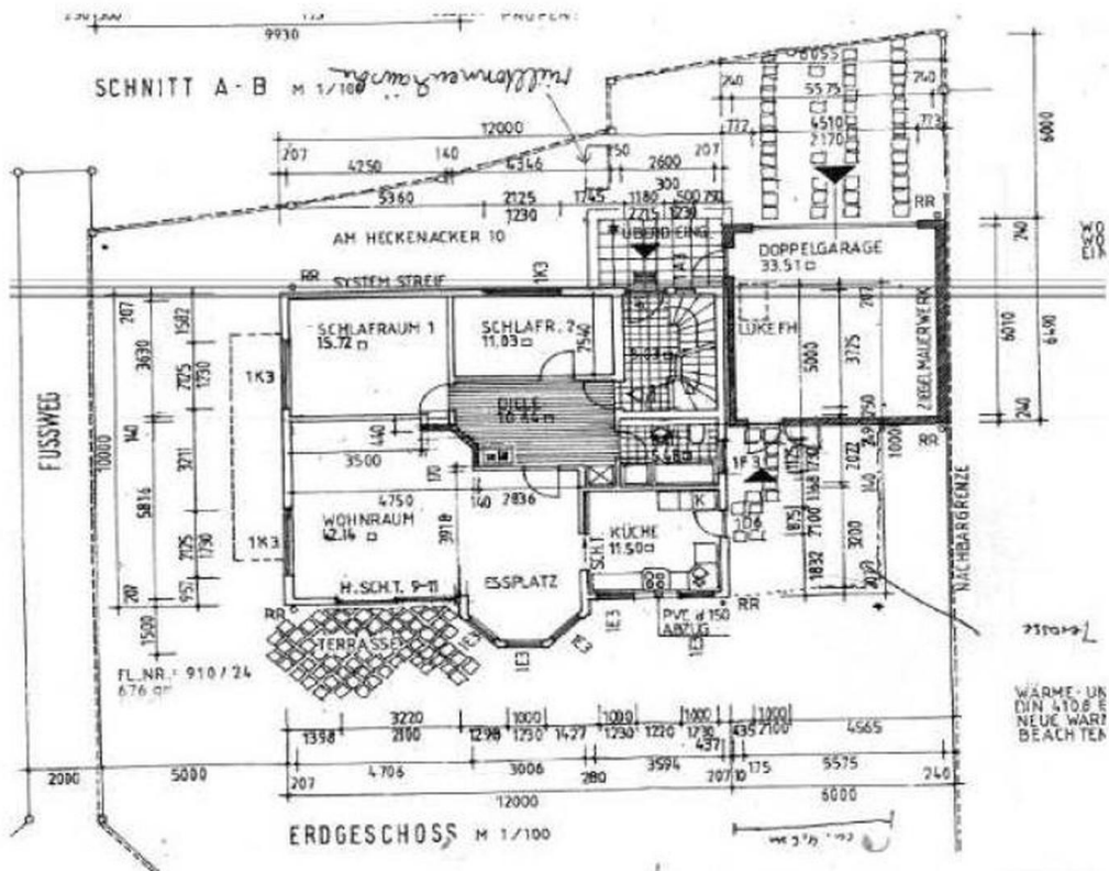
Grundriss Erdgeschoss
