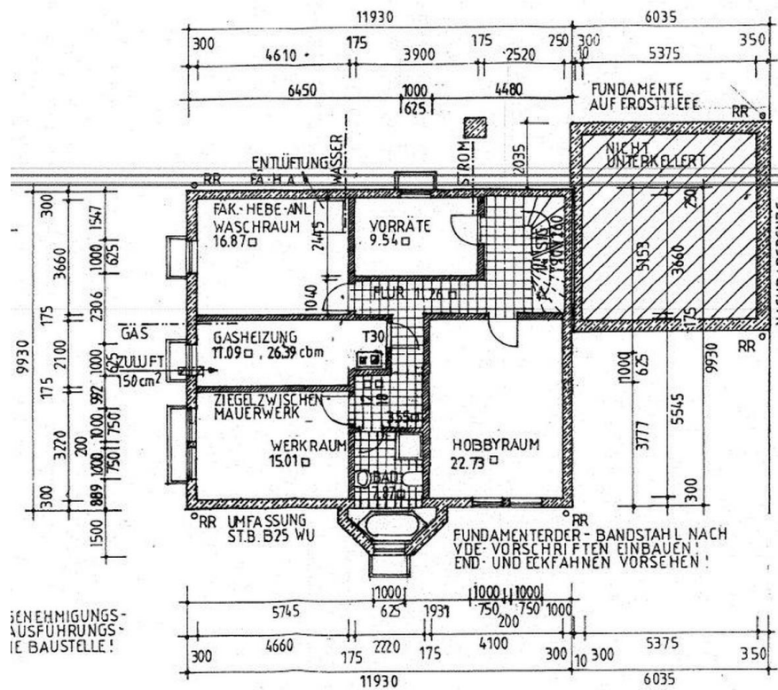
Grundriss Untergeschoss
