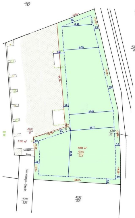
Grundstücksfläche mit Bemaßung
