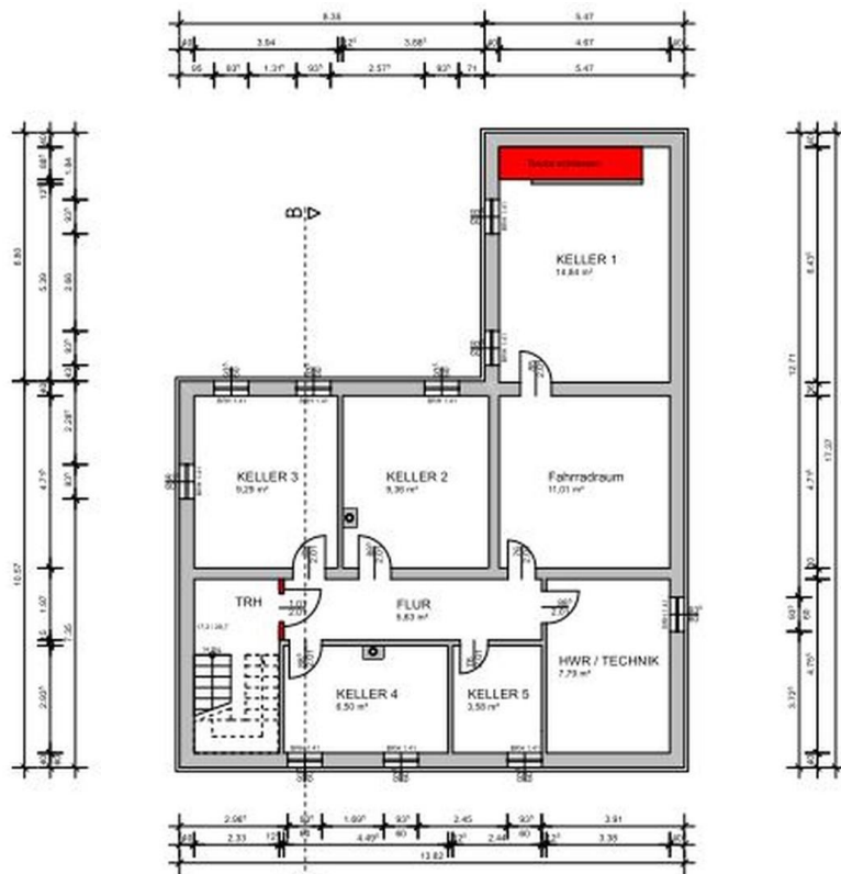
Grundriss Keller
