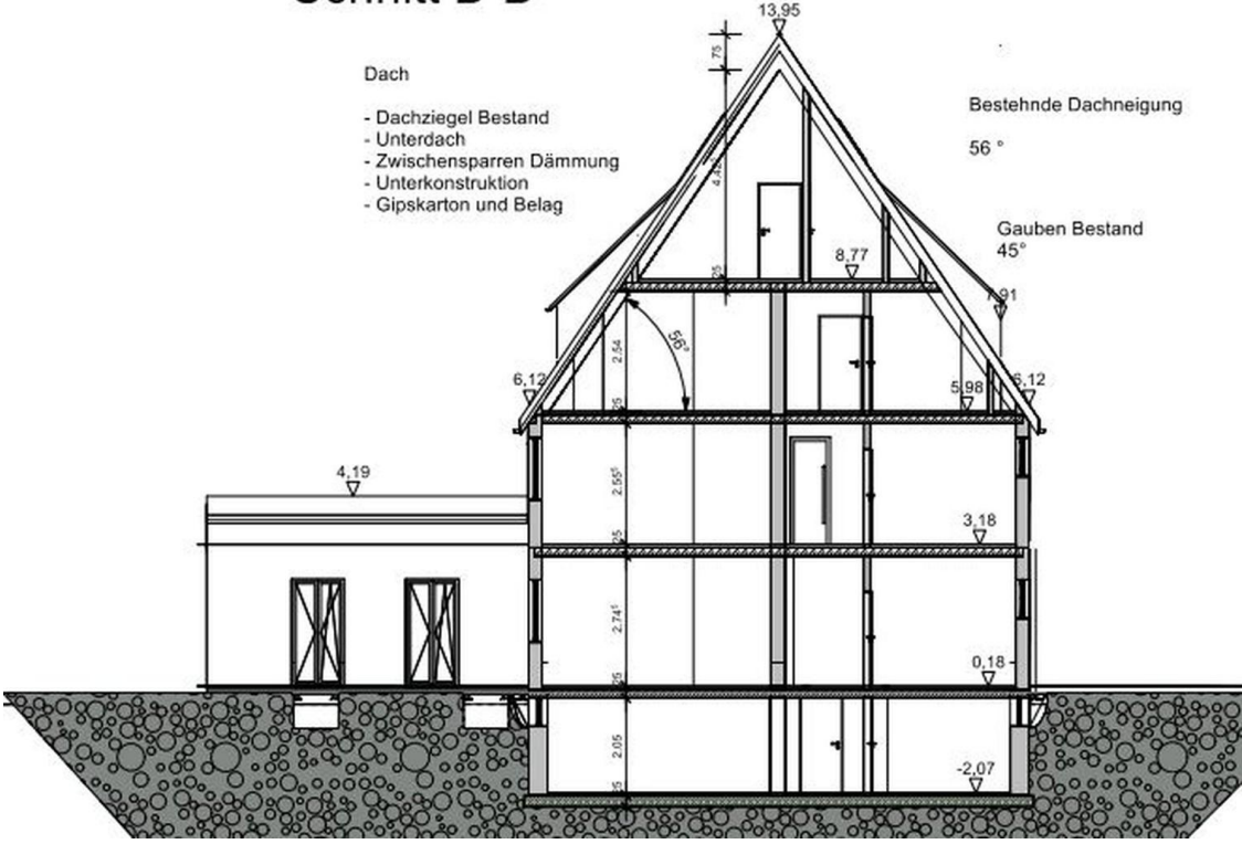
Schnitt
