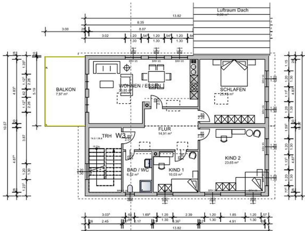
Grundriss 1.OG
