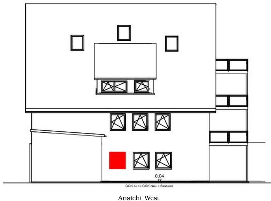
Ansicht von Westen M 1: 100
