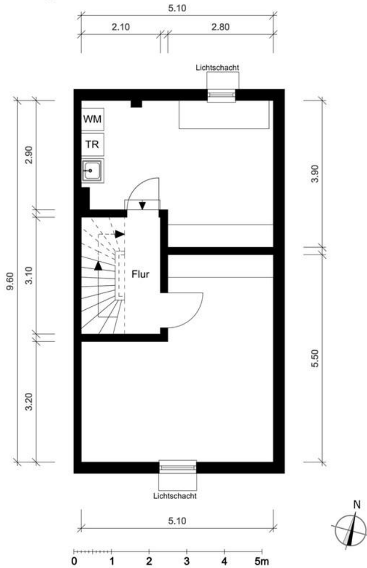
Kellergeschoss
