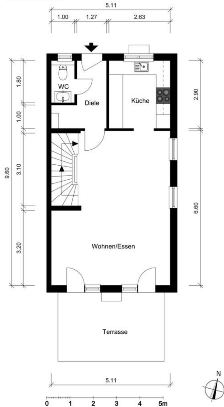
Erdgeschoss
