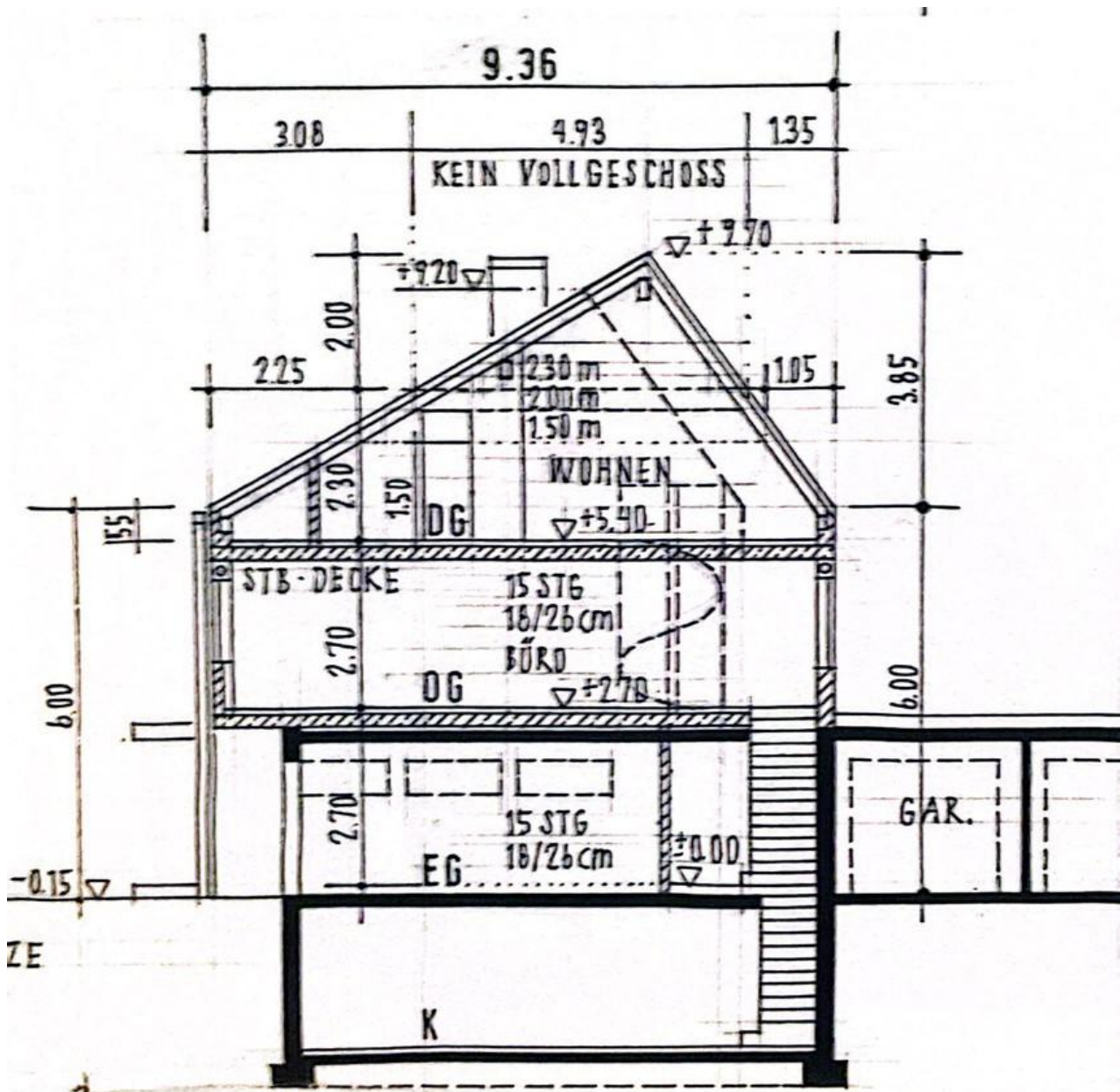
SCHNITT A-A
