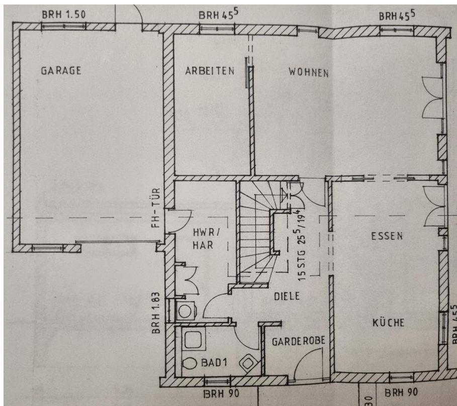
Erdgeschoss
