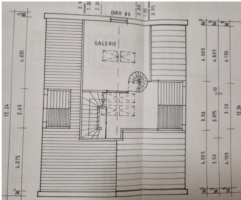
Dachgalerie
