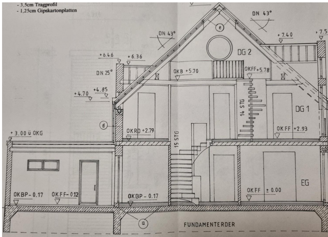
Schnitt
