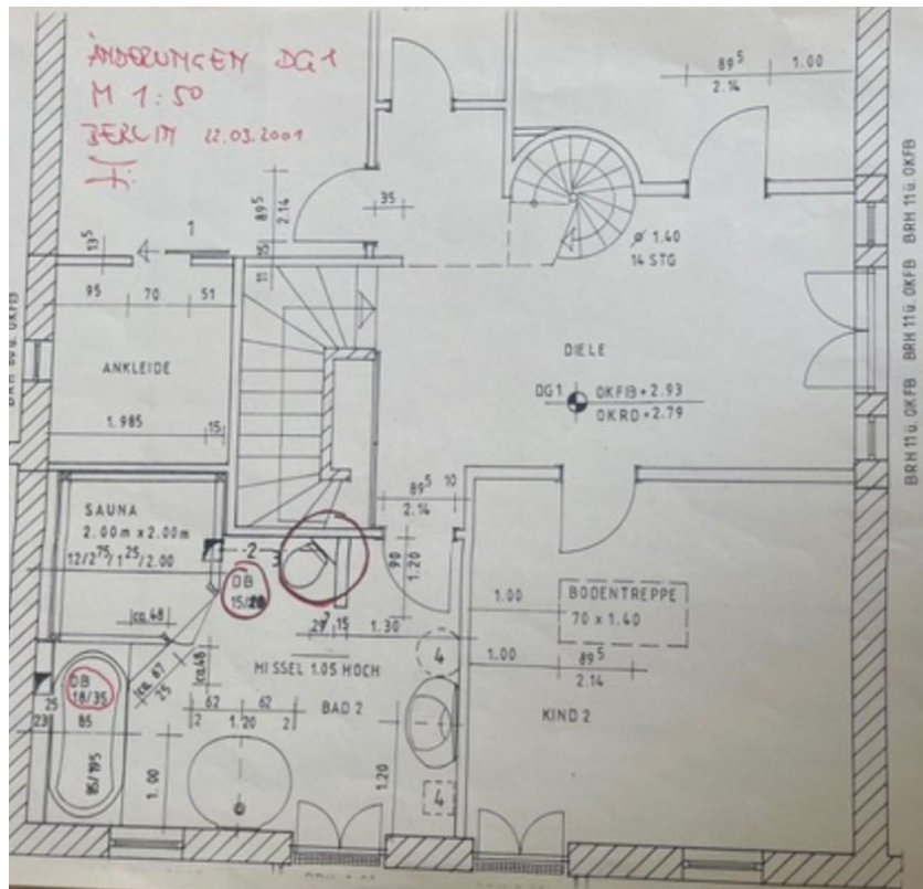
Obergeschoss
