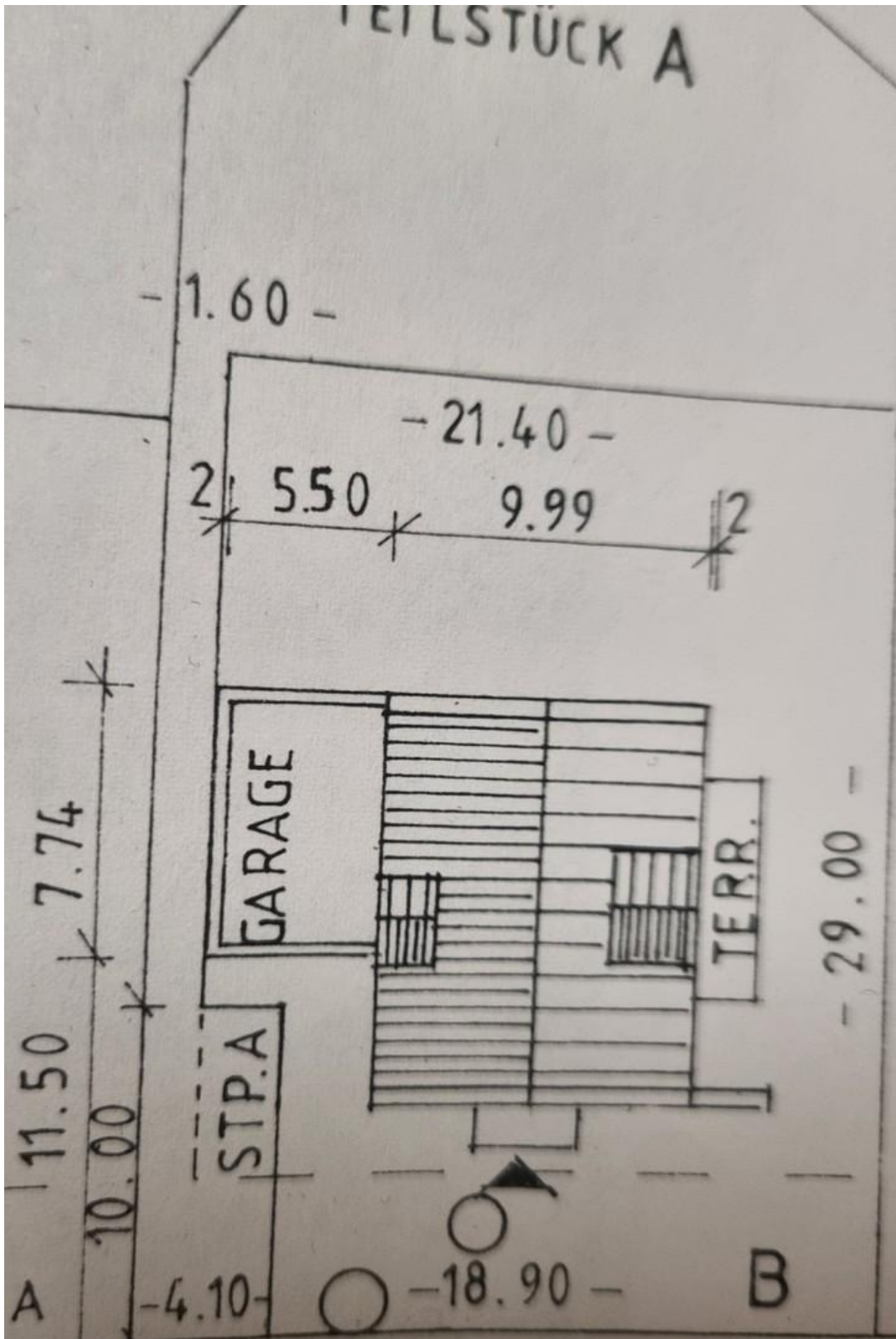
Draufsicht
