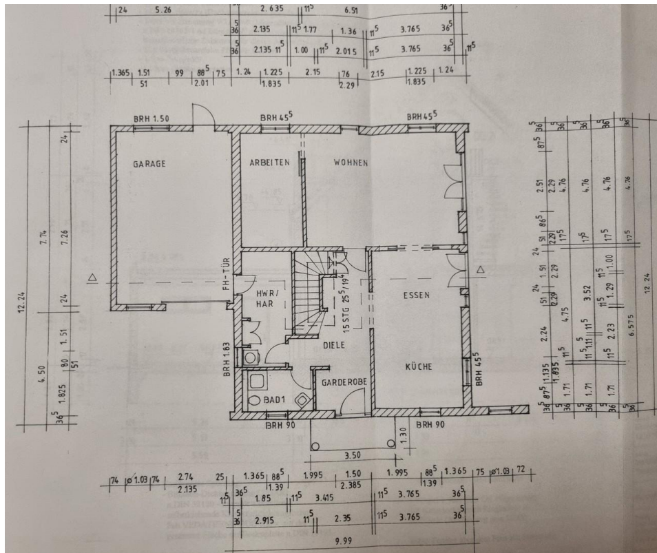
Erdgeschoss Bemaßung
