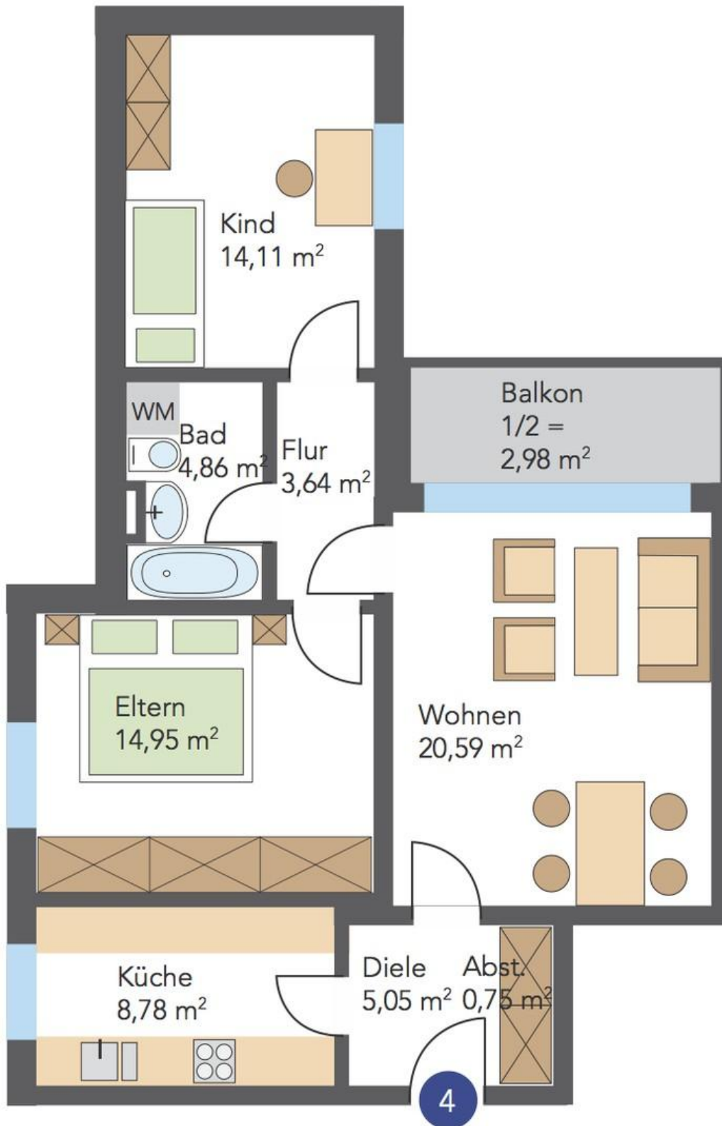
Grundriss
