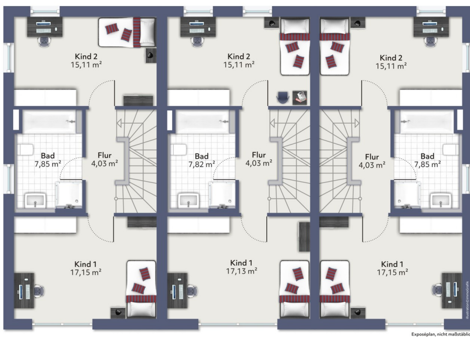
Obergeschoss
