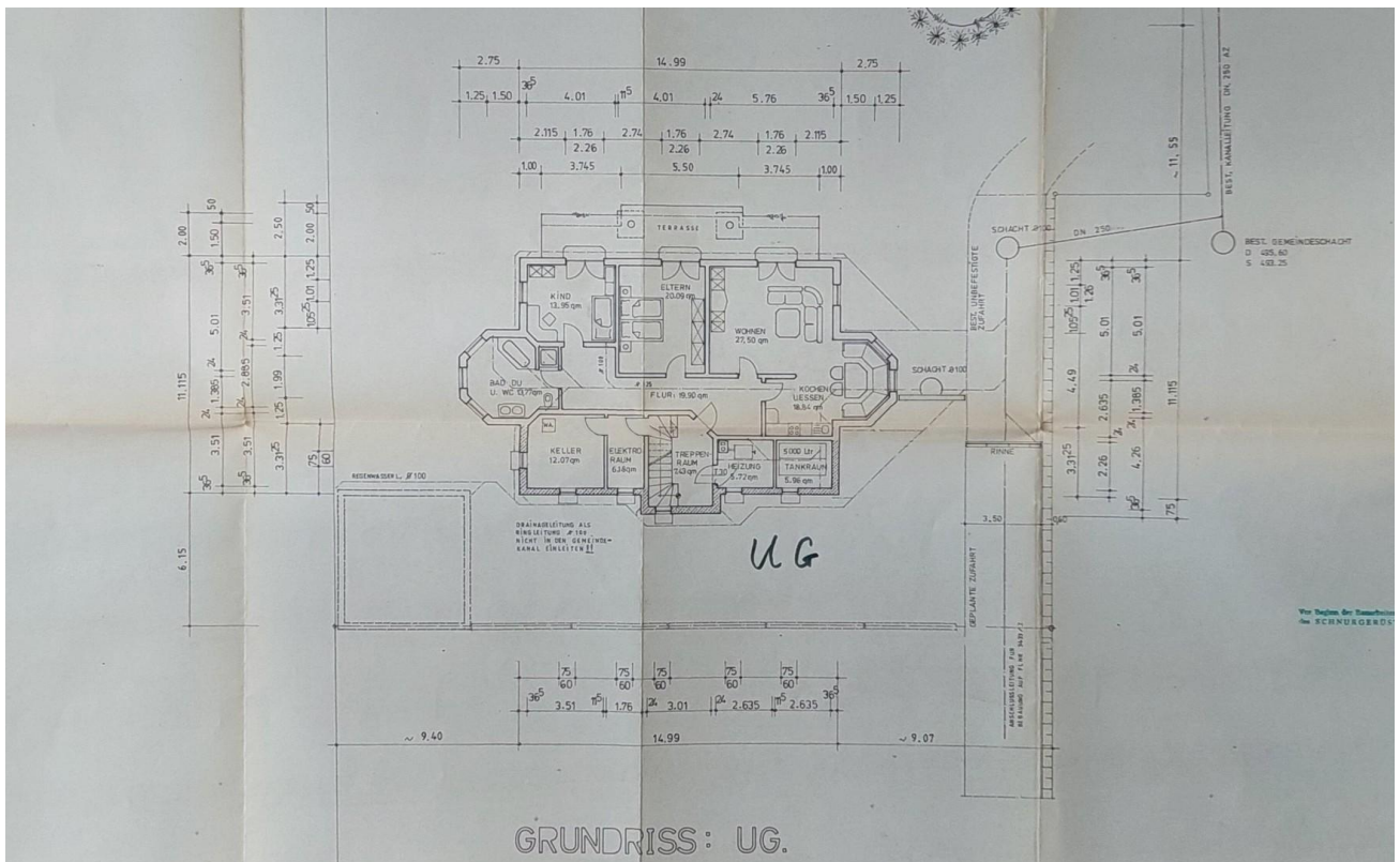
Grundriss Untergeschoss
