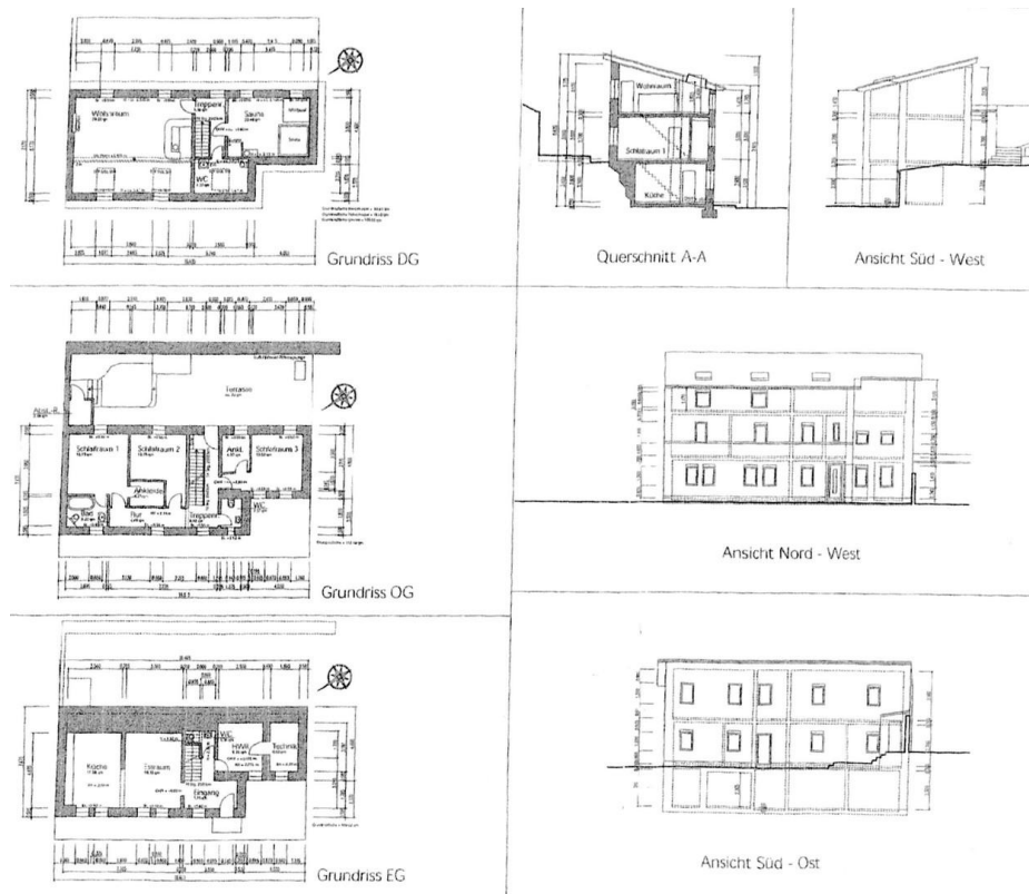
Grundriss/Hausansicht
