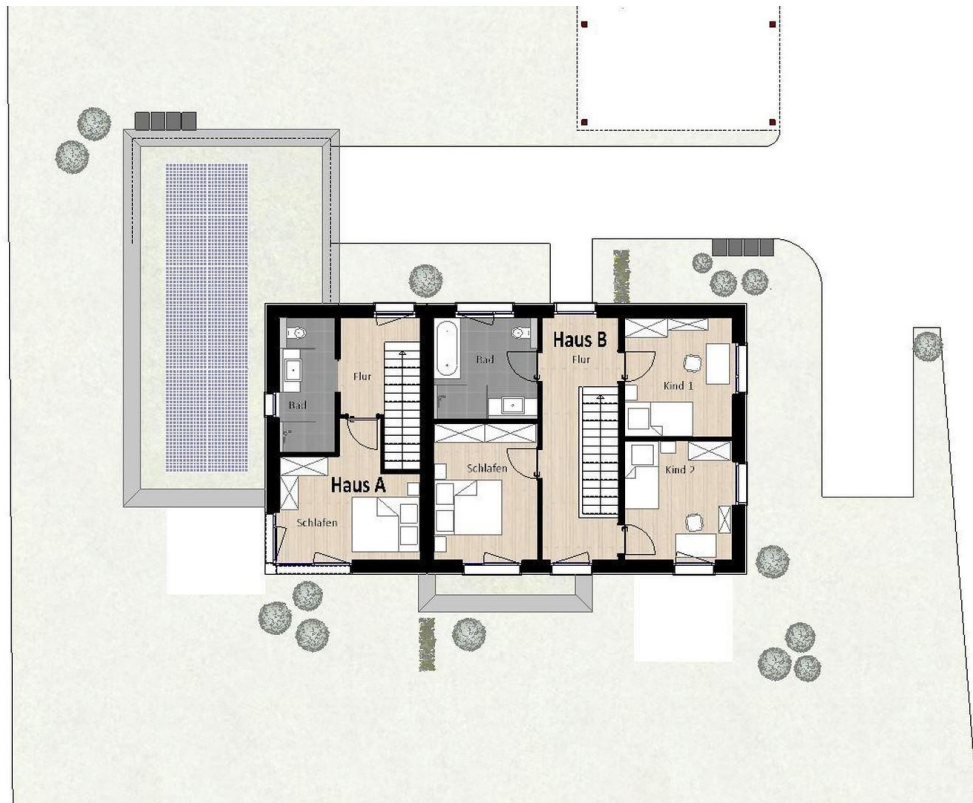
Doppelhaus 1 OG
