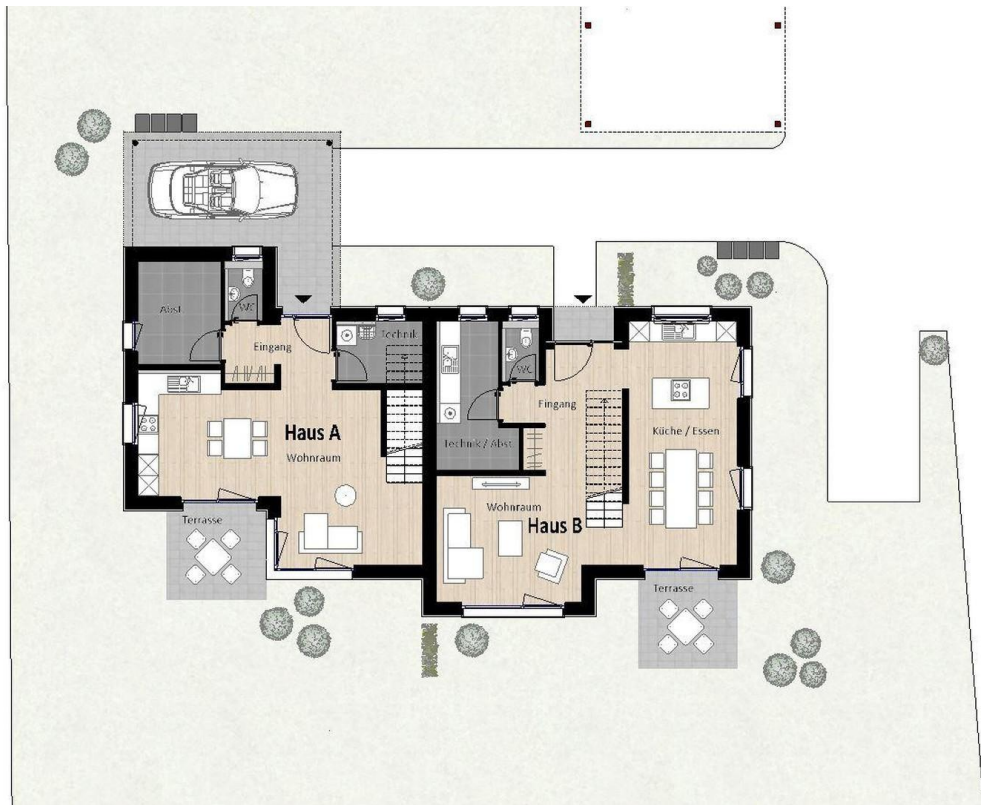
Doppelhaus 1 EG
