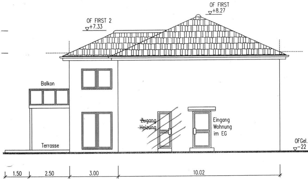
Ansicht von Norden - Eingangsfassade
