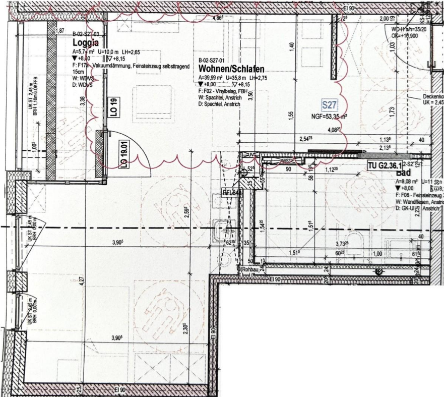
Grundriss
