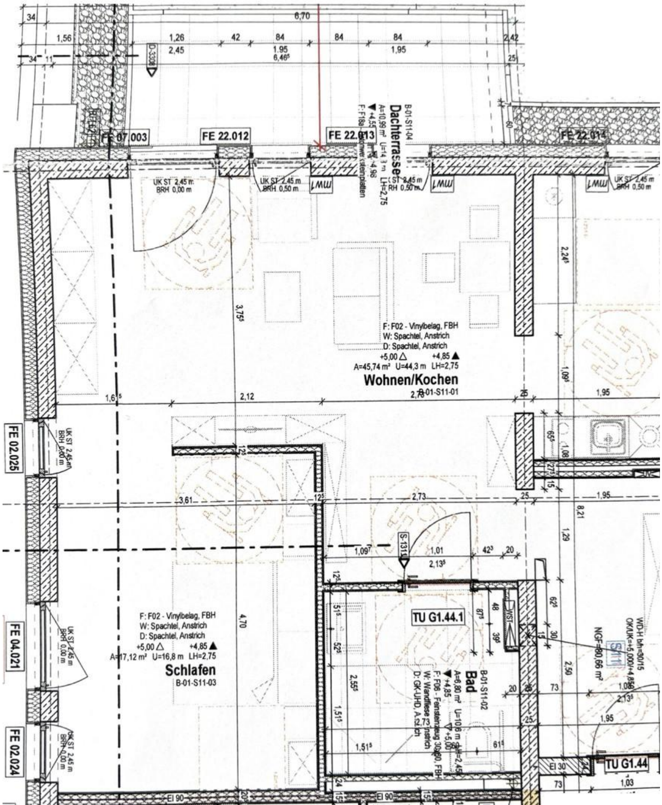
Grundriss
