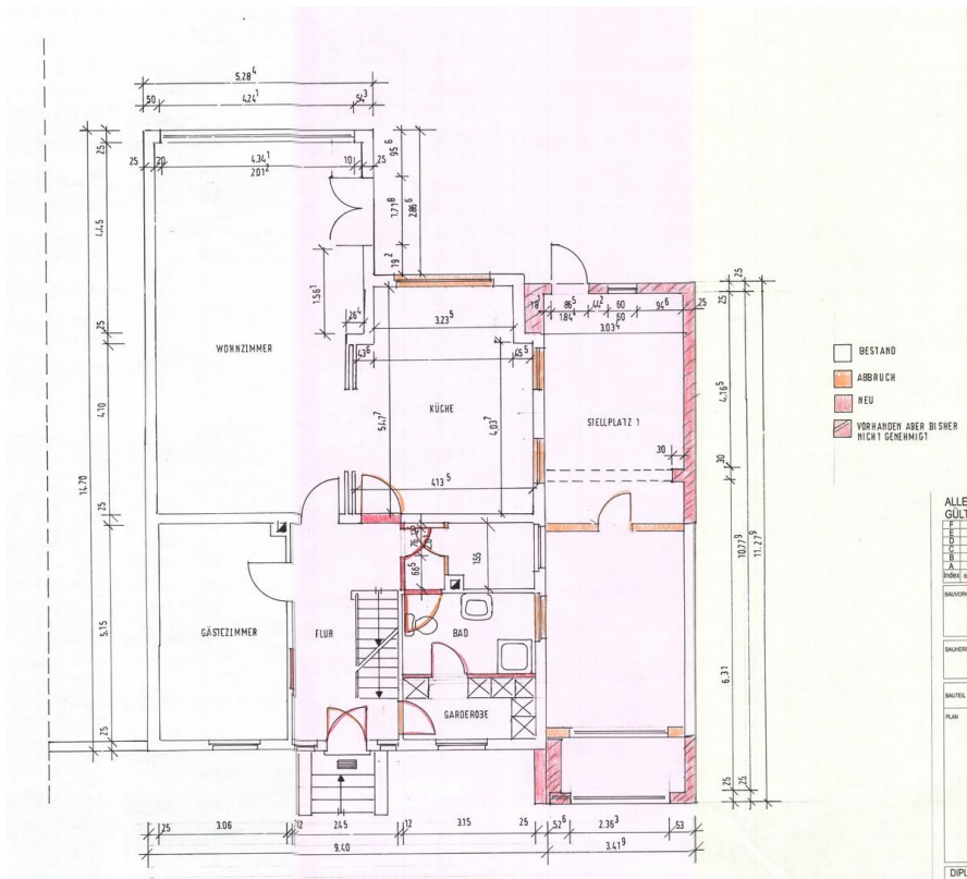
Grundriss EG
