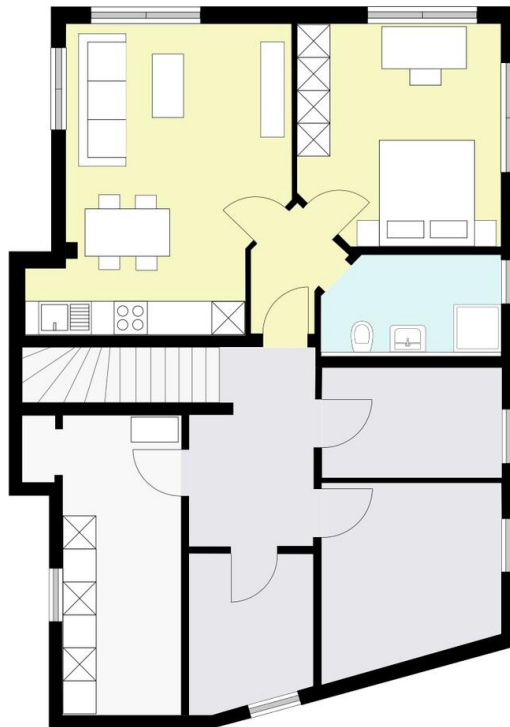
Grundriss UG
