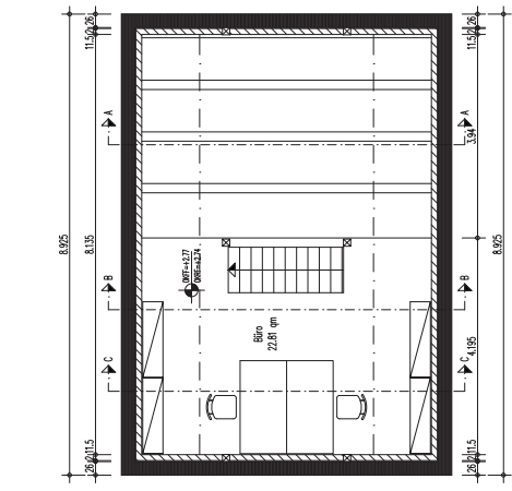
GRUNDRISS OBERGESCHOSS
