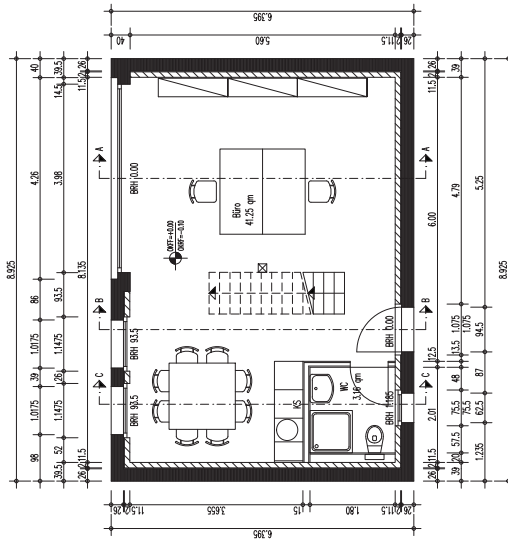
GRUNDRISS ERDGESCHOSS
