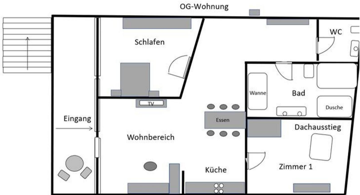
Grundriss
