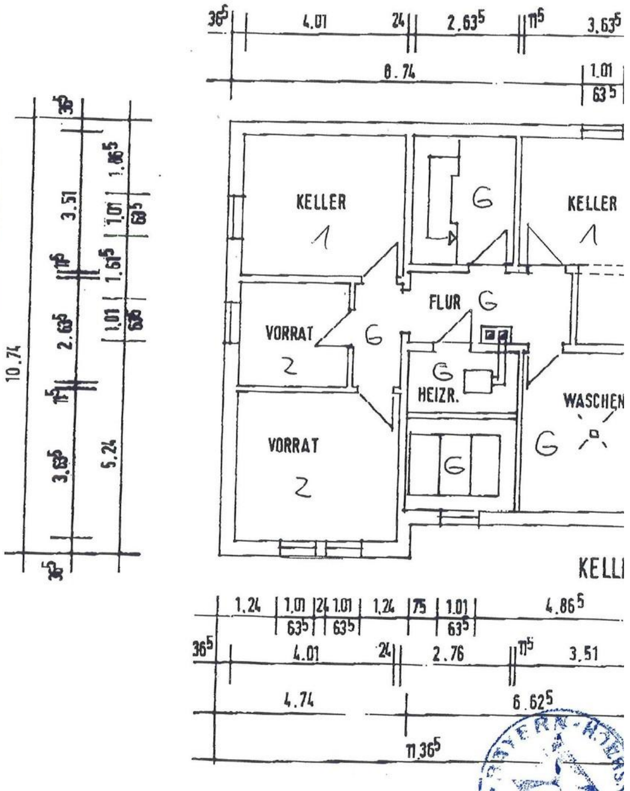
Grundriss - Kellergeschoss
