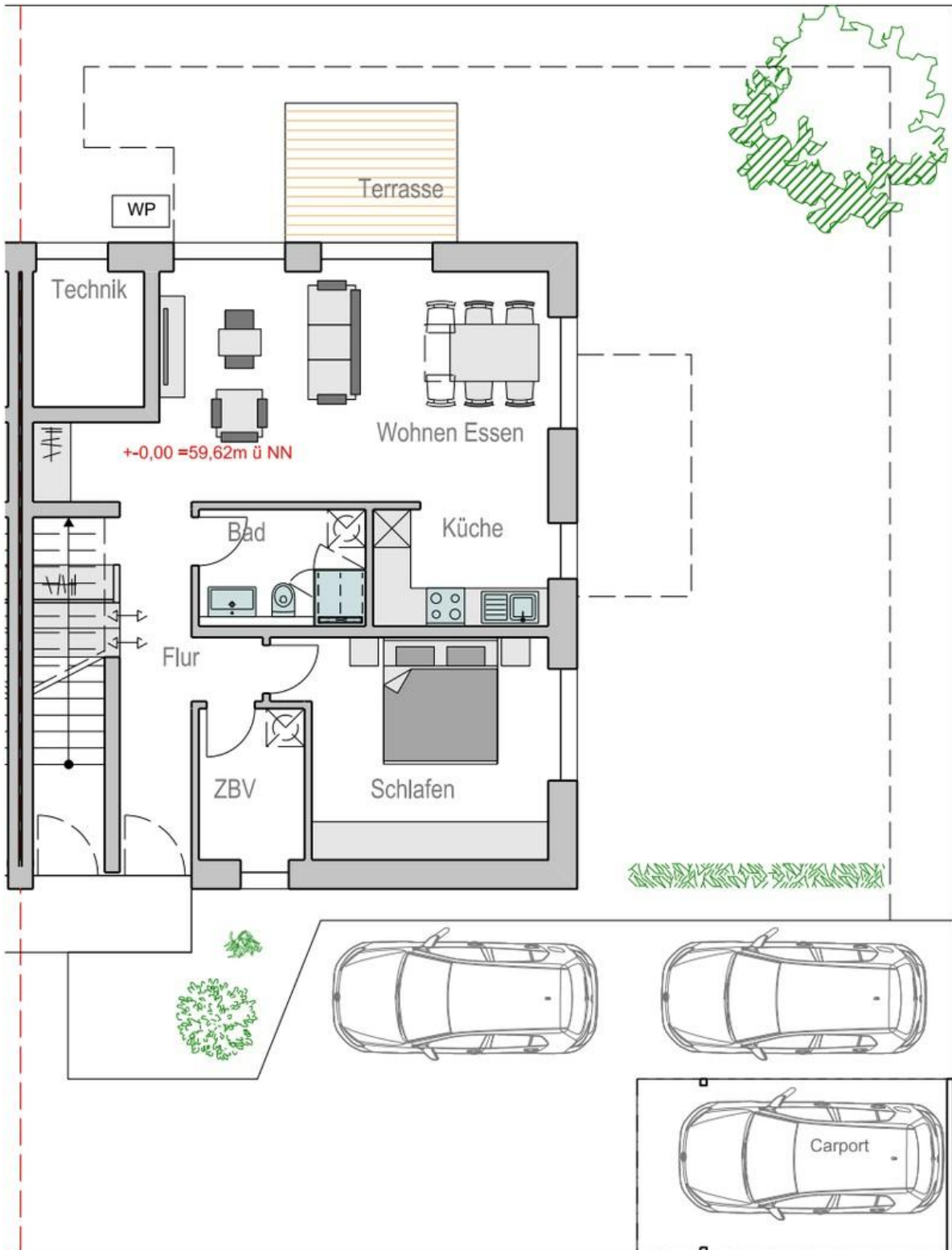
Erdgeschoss rechts
