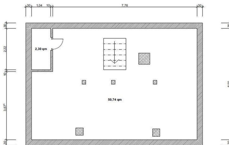
Dachspitz
