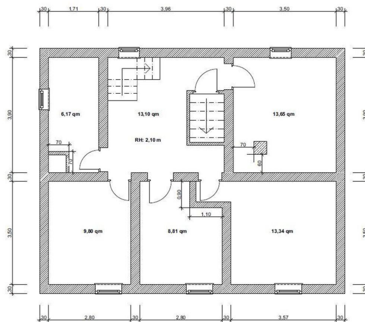
Obergeschoss
