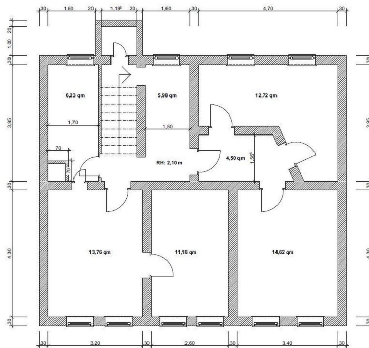
Dachgeschoss
