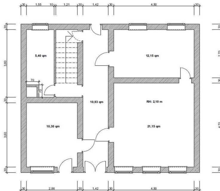
Erdgeschoss
