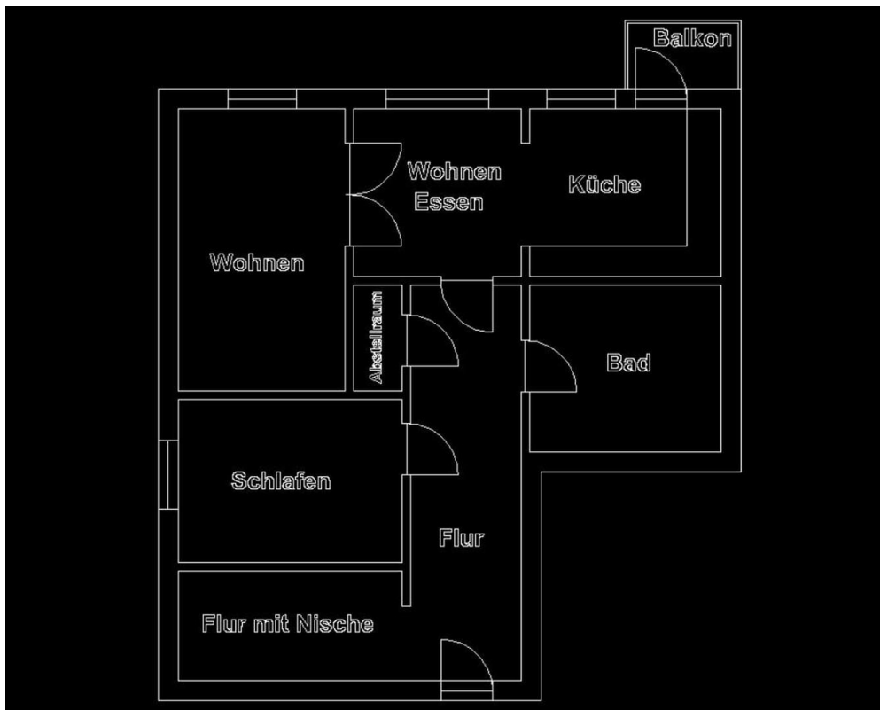
Grundriss-nicht maßstabgetreu
