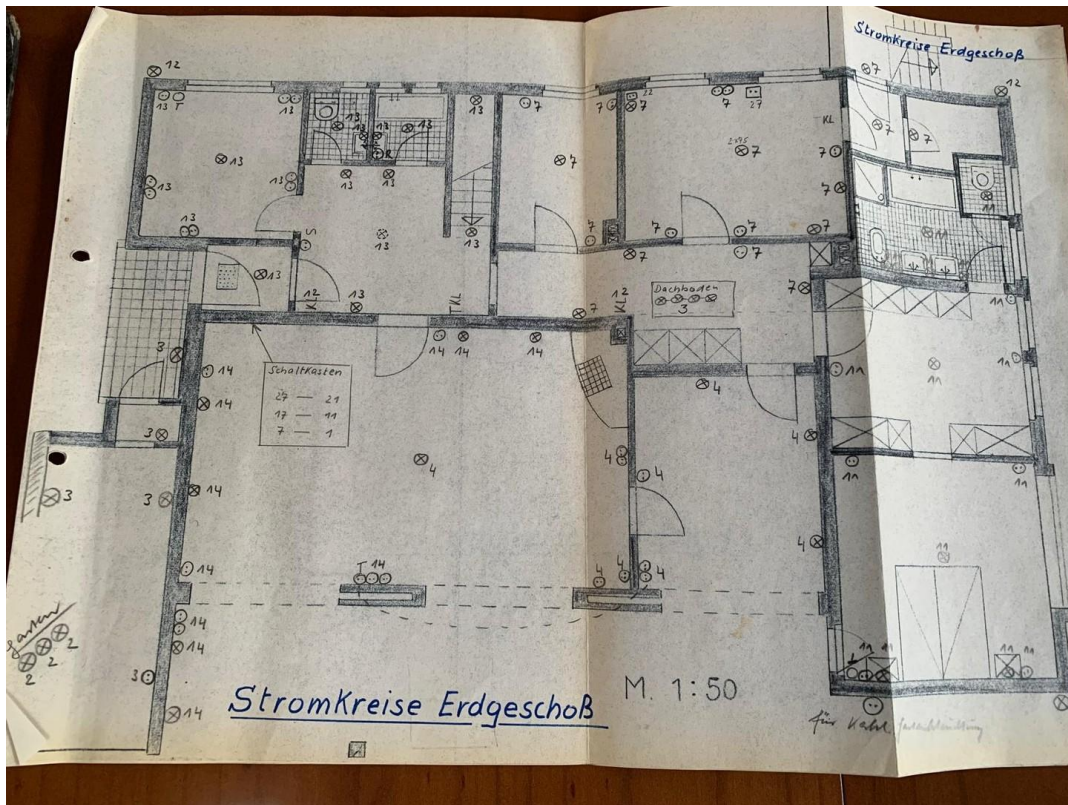
Grundriss Wohnbereich
