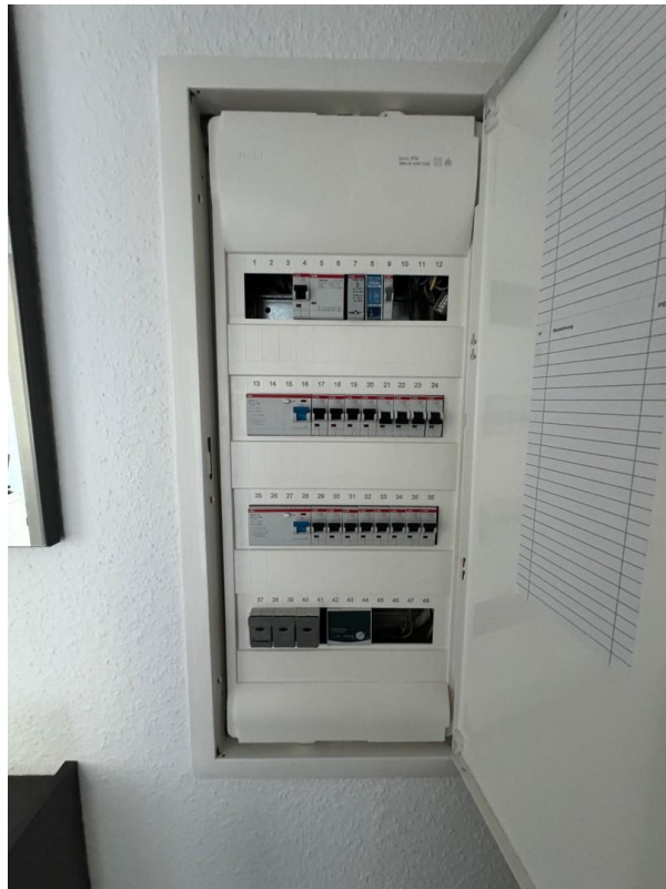
Elektrokasten
