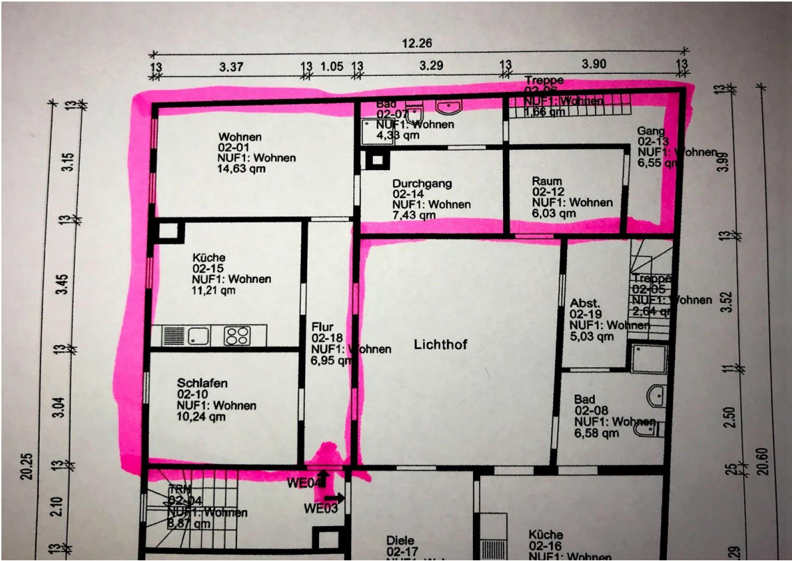
Grundriss JPG
