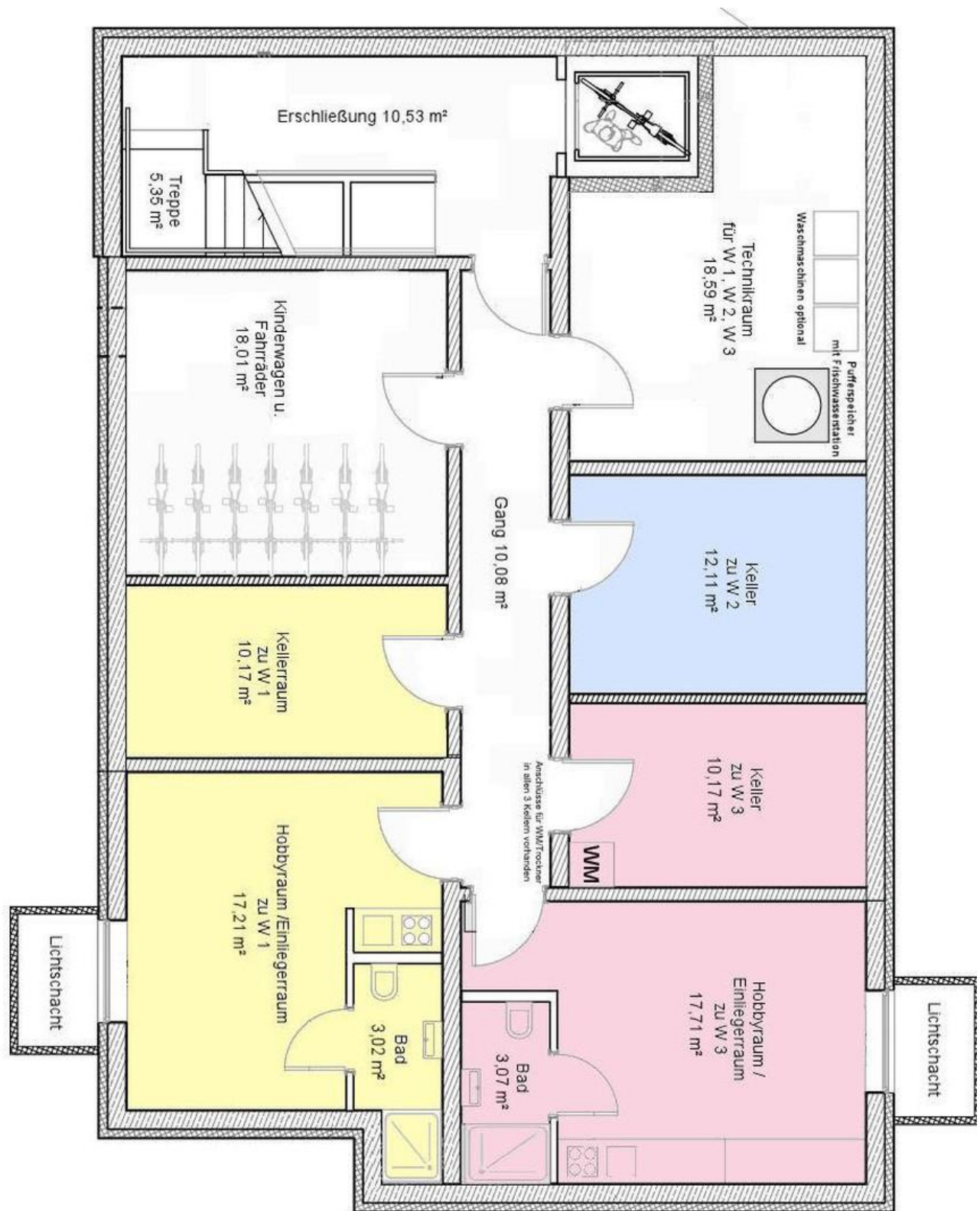
Grundriss Untergeschoß
