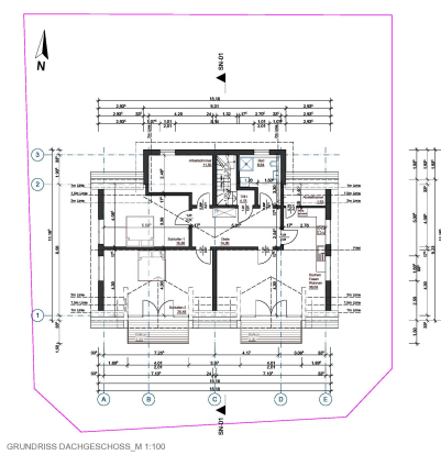
GRUNDRISS DACHGESCHOSS_M 1:100
