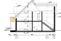
SCHNITT 1-1_M 1:100
