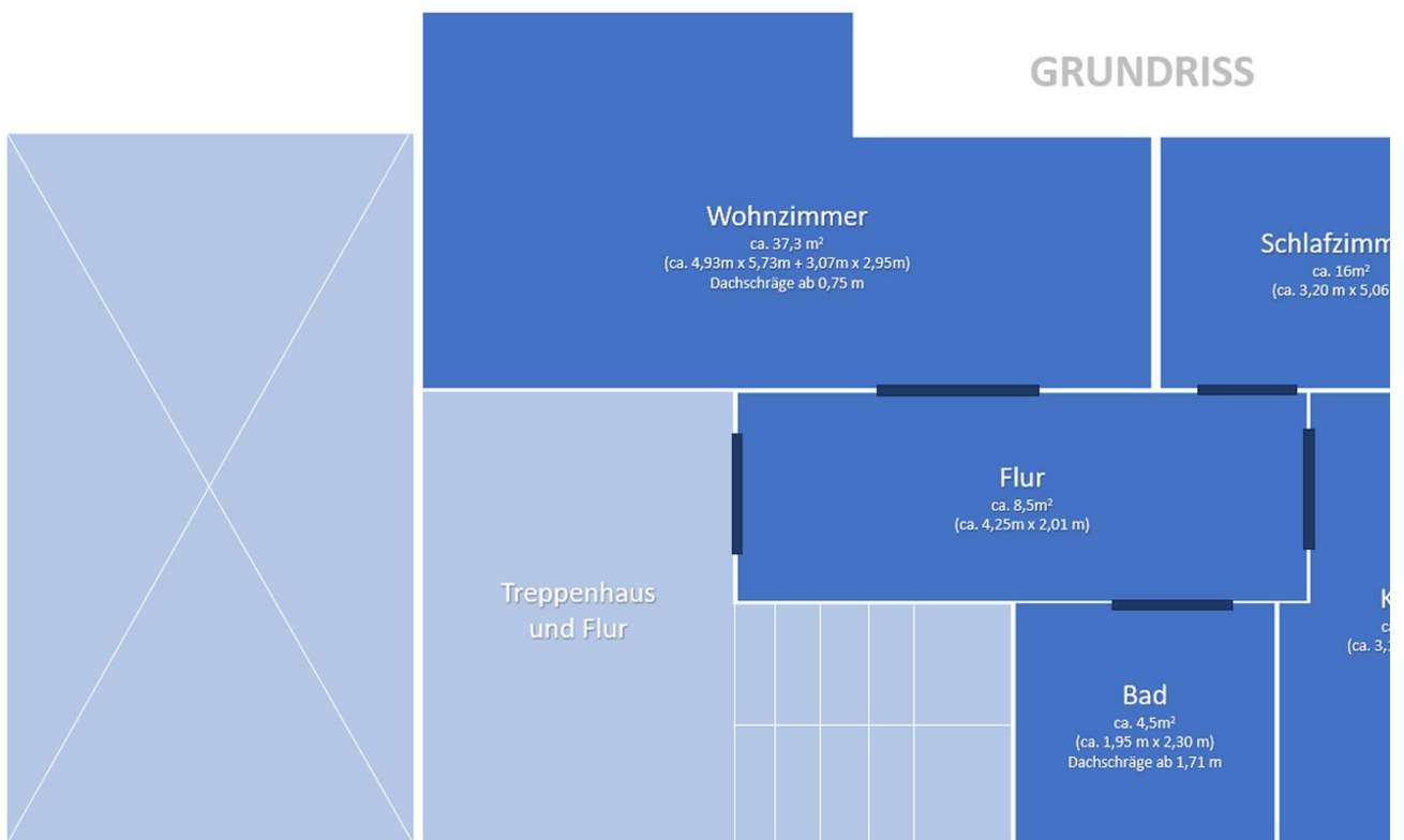
Grundriss
