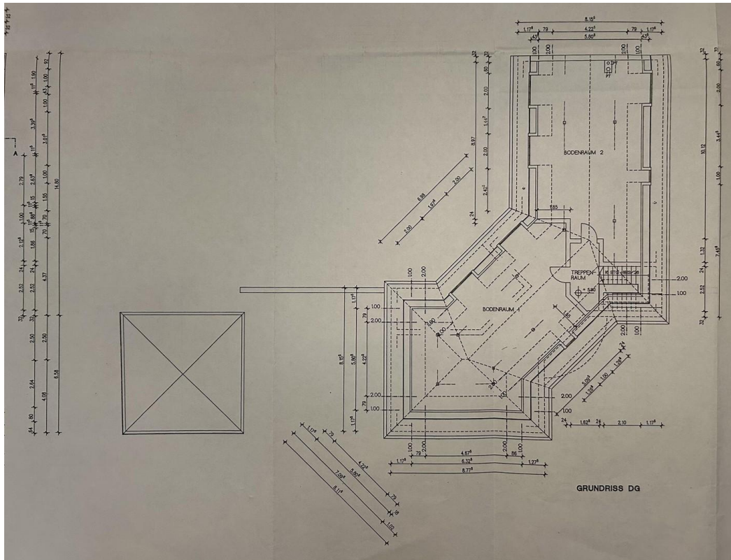
Dachgeschoss
