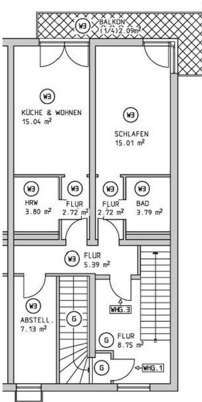
Grundriss
