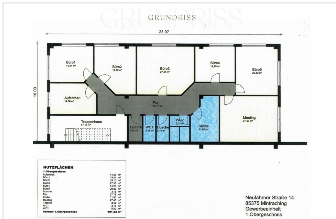
Grundriss
