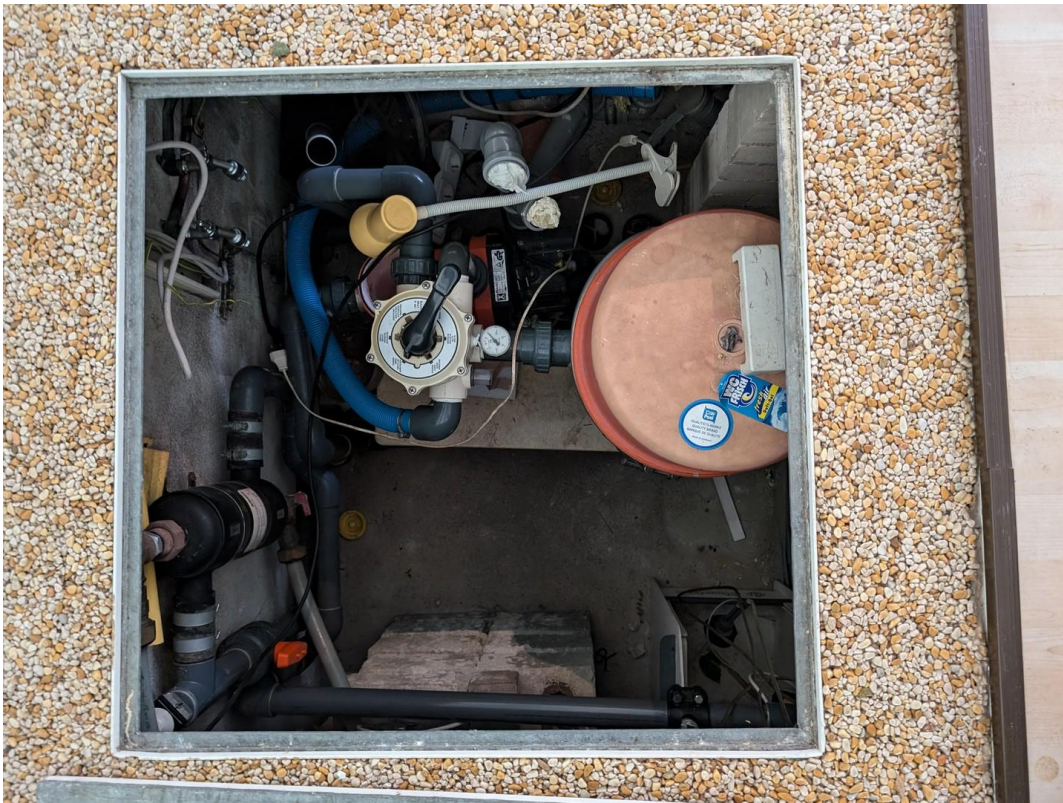
Gegenstromanlage und Filter
