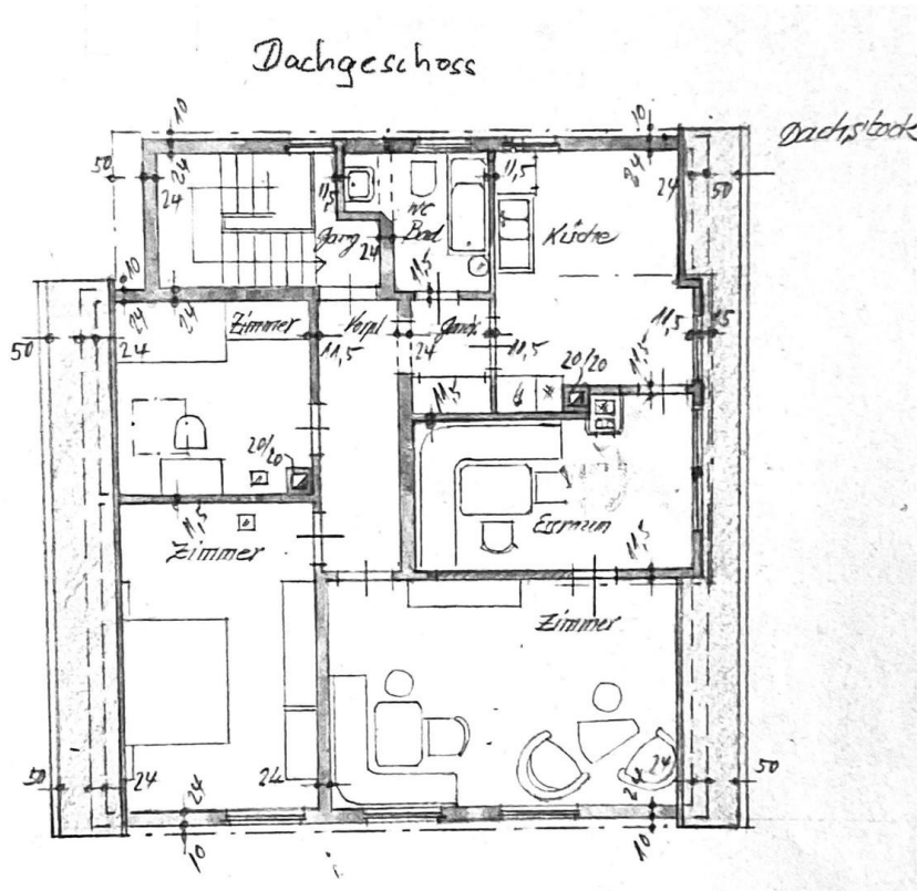
Grundriss Dachgeschoss
