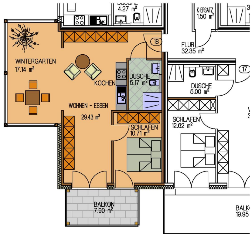
Wohnung № 18 1. OG
