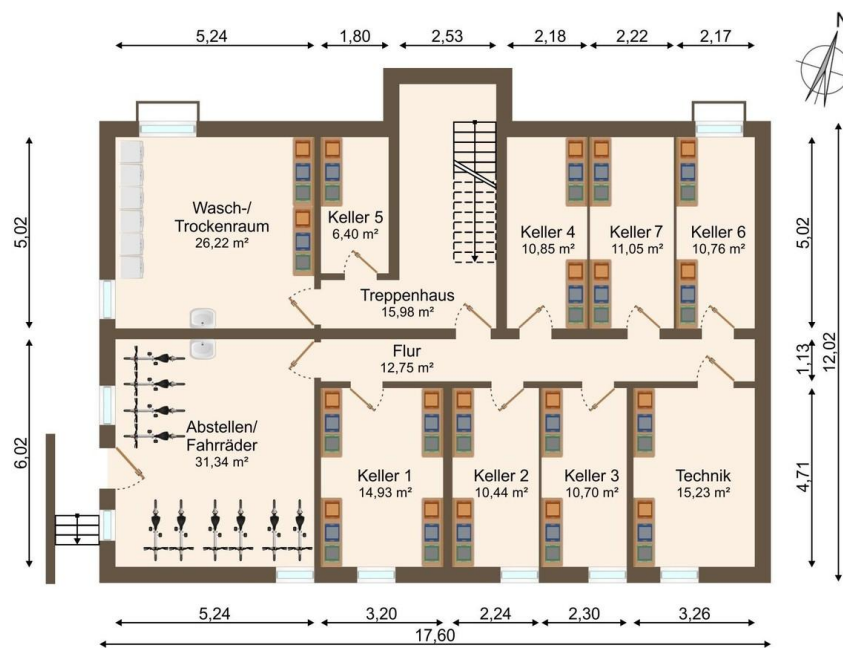
Grundriss Keller 7
