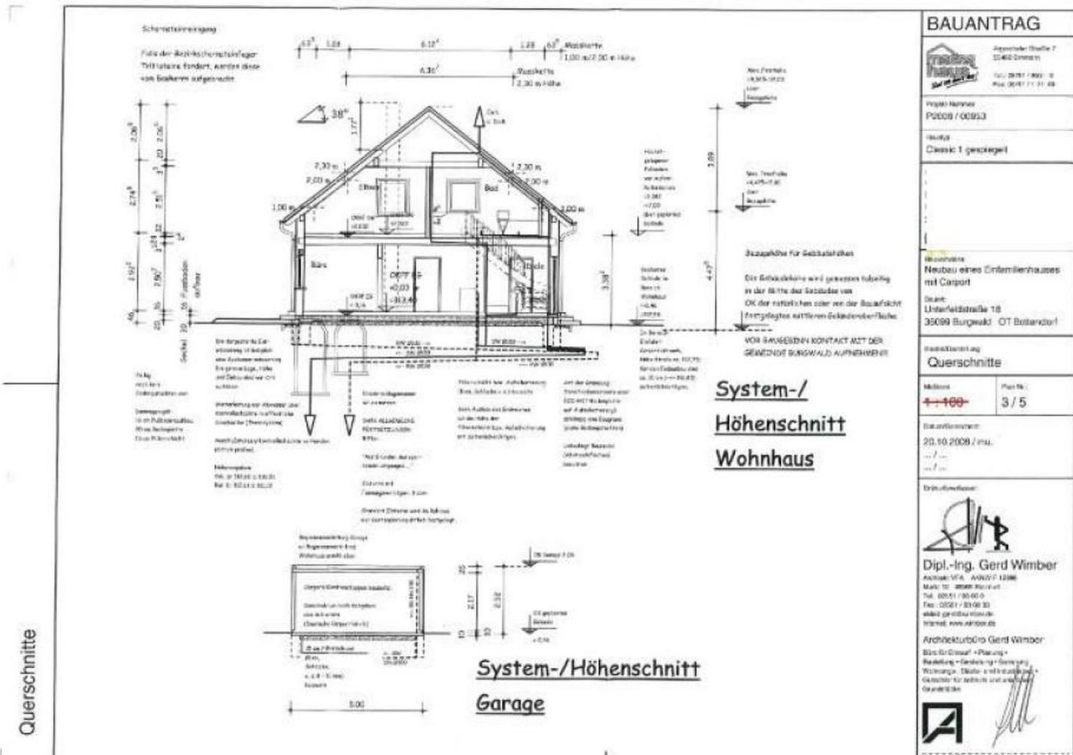
Schnitt
