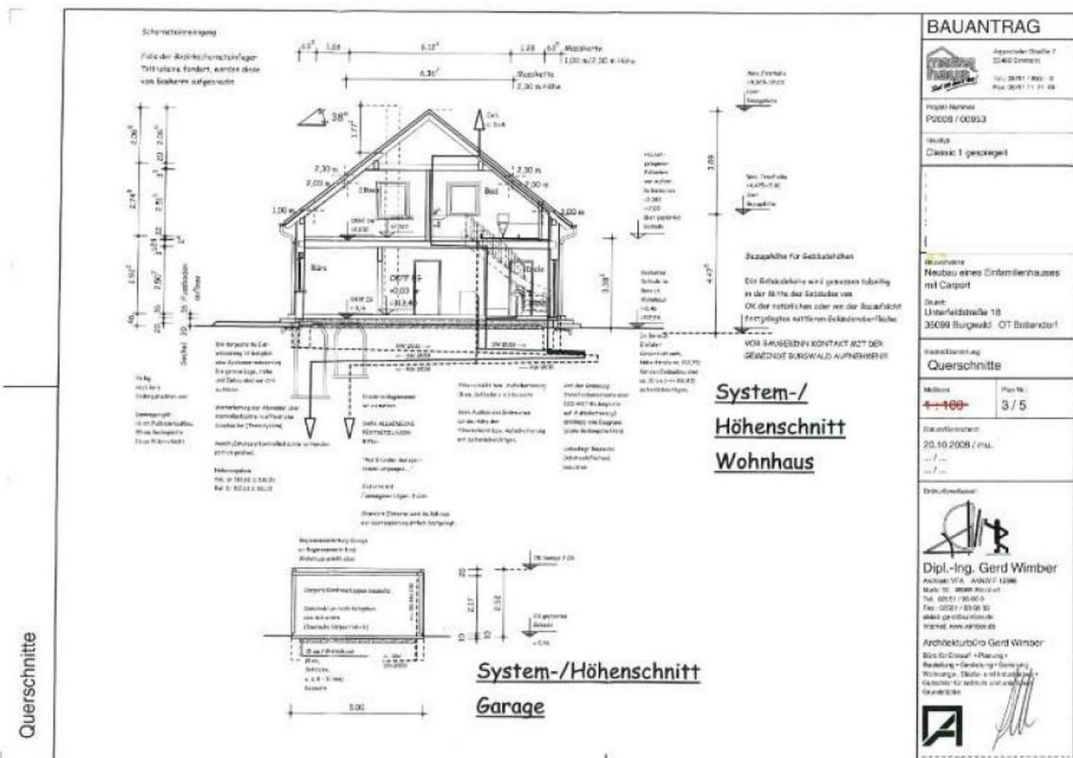
Schnitt
