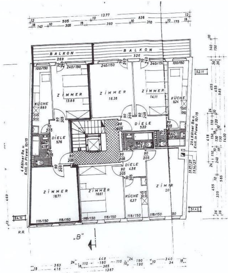
1.-4. OBERGESCHOSS
