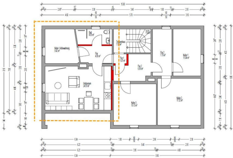
Grundriss Kellergeschoss
