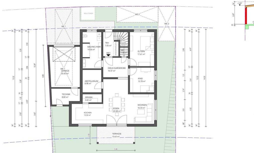
Marien Höhe - 2-Fam.H. - GrundrisseSchnitte_3_938233_7,0.pdf 396 KB
