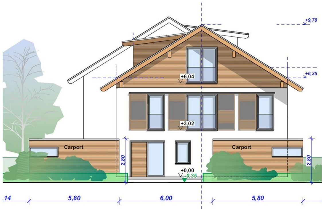
Straßenansicht Vorplanung
