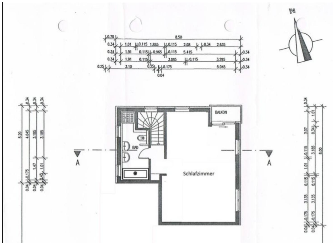
Grundriss 1.OG
