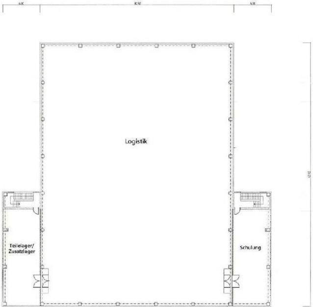
2. Obergeschoss
